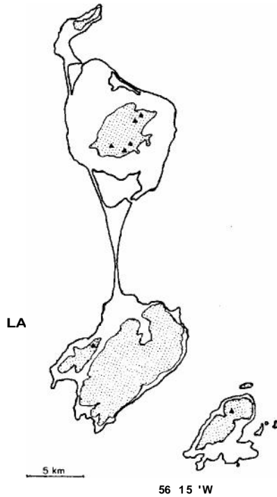
FIG. 3. Topographie des îles St-Pierre et Miquelon. Les régions en pointillé ont une altitude supérieure à 100 m. Les triangles représentent les sommets de plus de 200 m.
